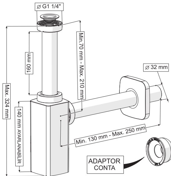
250 mm QUAD SİFON TAŞMA DELİKSİZ ELIXIR POP-UP
